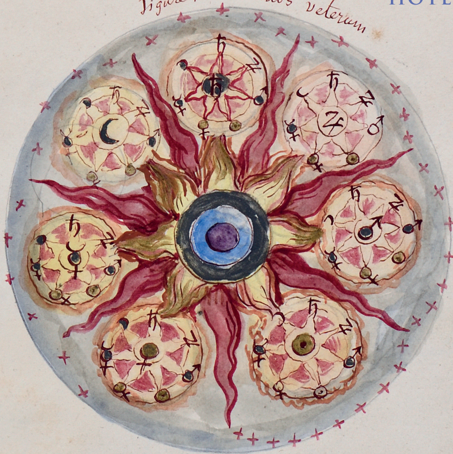
figure 11 Subiectum chymicum
